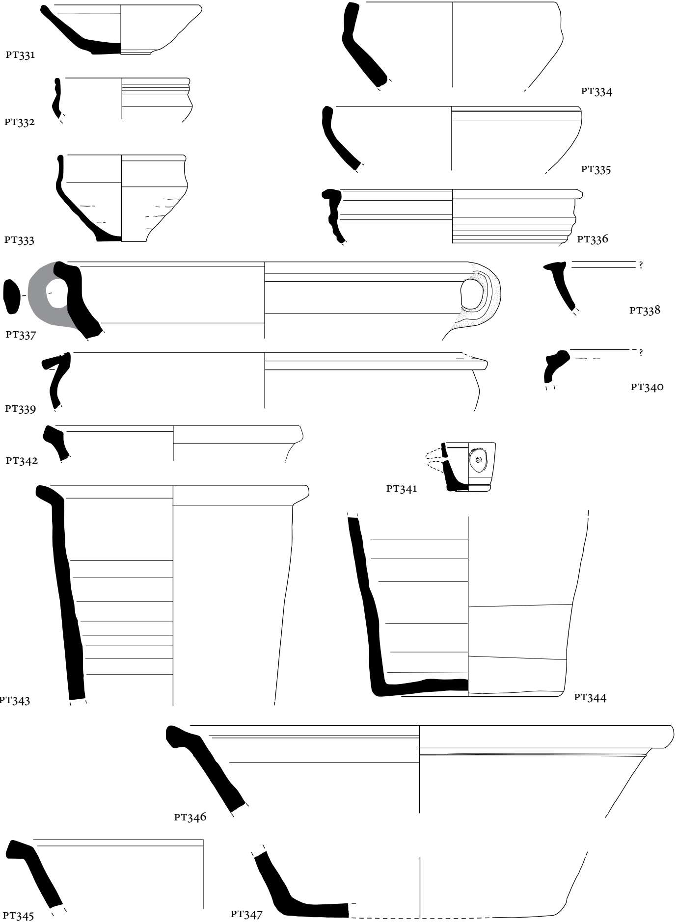
Plate 19. Group D. Buff wares 1-3 (PT331-347). Scale 1:3.
