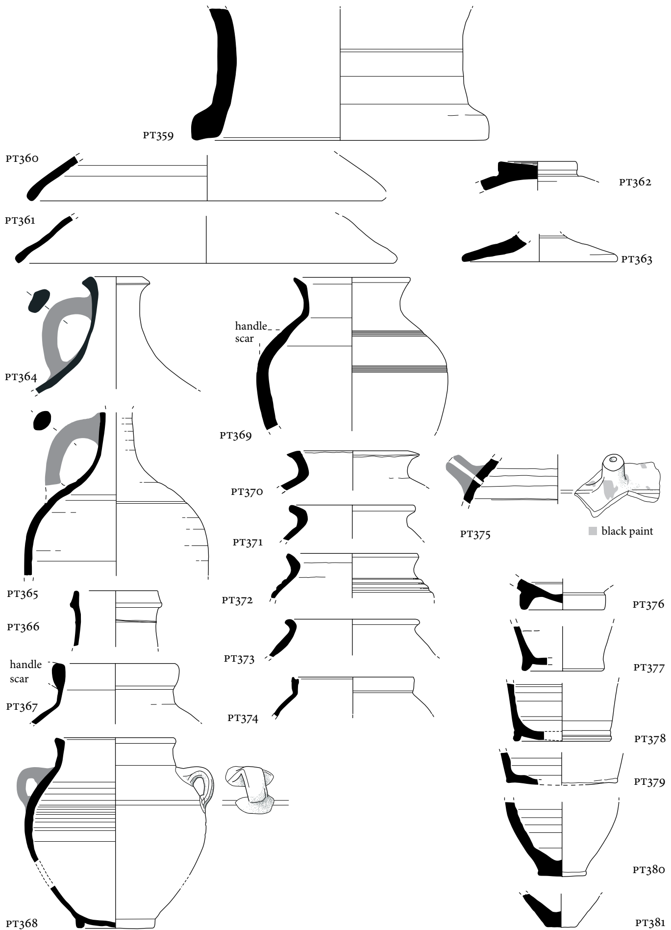
Plate 21. Group D. Buff wares 1-3 (PT359-381). Scale 1:3.
