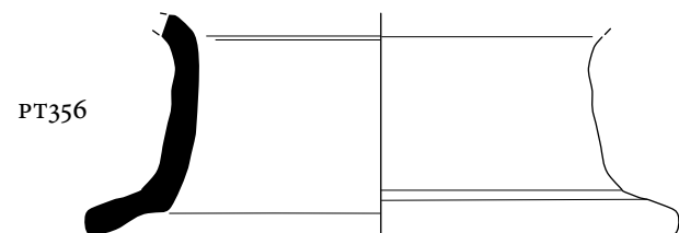
Plate 20. Group D. Buff wares 1-3 (PT348-358). Scale 1:3.
