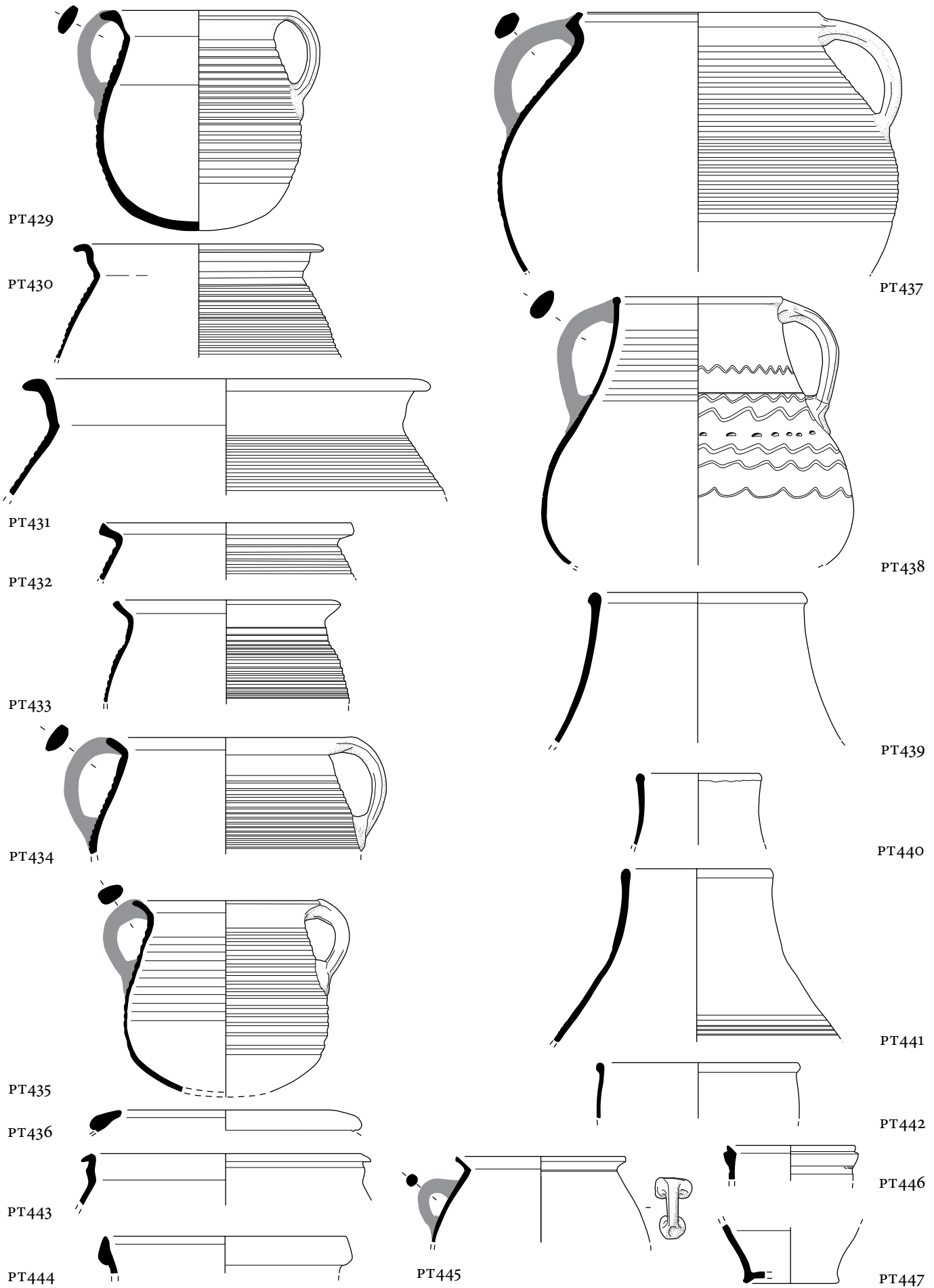
Plate 27. Group D. Cooking ware 1 (PT429-447). Scale 1:3.
